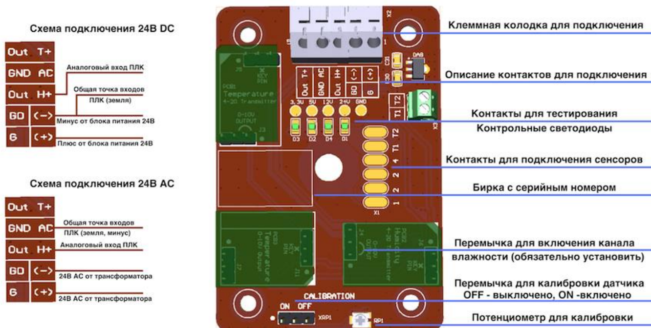
Табл. 2 Подключение датчика влажности, схема соединений и описание
